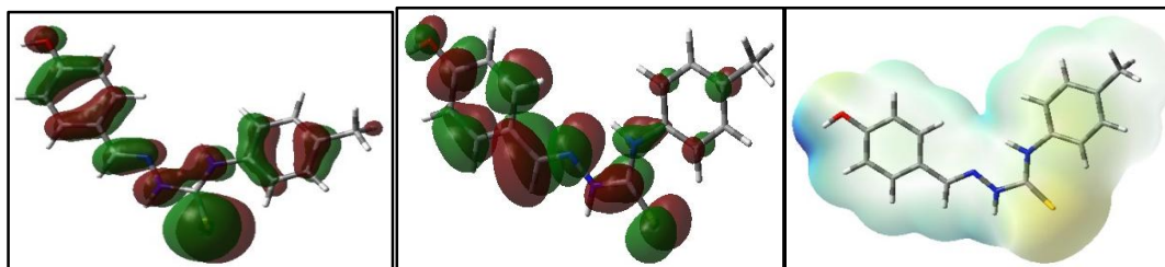
Molecule 15-HOMO
