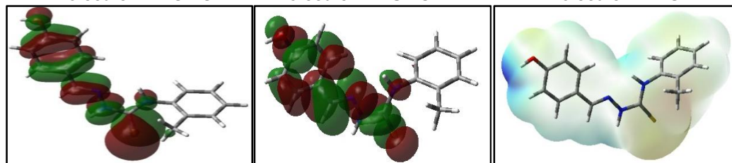
Molecule 13-HOMO
